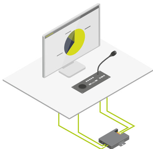
Configurazione di uniBOX PRO con uno schermo da tavolo e un'unità con montaggio a filo con moduli Confidea a scelta
