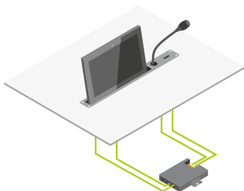
Configurazione di uniBOX PRO con schermo motorizzato
