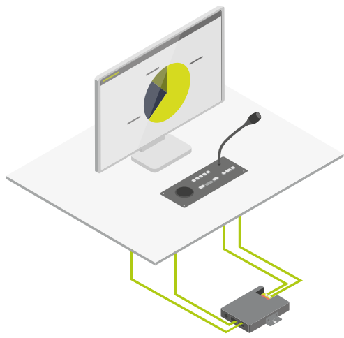
Configuration uniBOX PRO avec écran sur table et unité encastrée avec les modules Con idea de votre choix
