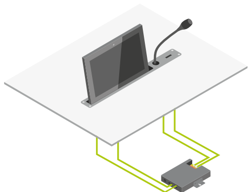
Configuration uniBOX PRO avec écran motorisé
